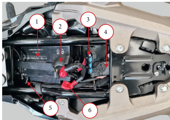
Фото 3.1. Аккумуляторный отсек: 1 – аккумуляторная батарея (АКБ); 2 – реле стартера; 3 – блок с предохранителями; 4 – модуль управления; 5 – защитный колпачок отрицательной («-») клеммы АКБ; 6 – защитный колпачок положительной («+») клеммы АКБ.
