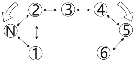
Рисунок 2. Схема переключения передач.
