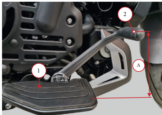
Фото 2.20. Регулировка педали тормоза:
