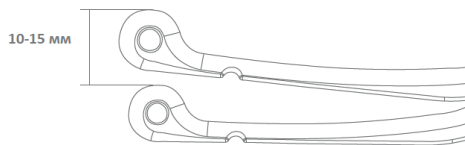
Рисунок 1. Свободный ход рычага сцепления.
