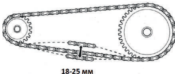
Рисунок 3. Натяжение цепи.
