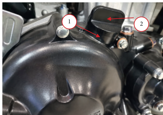
Фото 2.25. Доливание масла:
