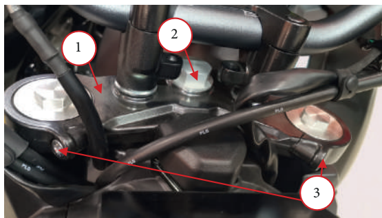
Фото 4.15. Регулировка подшипников рулевой колонки:
