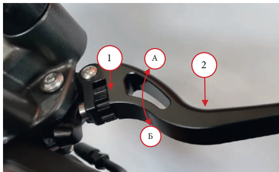
Фото 2.15. Регулировка рычага тормоза: 1 – регулировочная гайка; 2 – рычаг тормоза.
