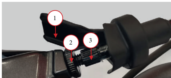
Рисунок 1. Свободный ход рычага сцепления.
