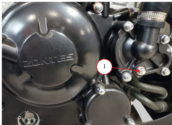
Фото 4.8. Слив охлаждающей жидкости: 1 – болт слива жидкости.
