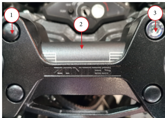
Фото 2.14. Крепление руля: 1 – пластиковые заглушки (4 штуки); 2 – руль; 3 – крепежные болты (4 штуки).
