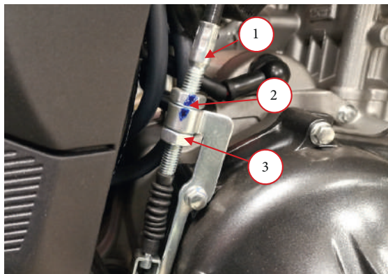
Фото 2.19. Регулировка сцепления на двигателе: 1 – регулятор; 2 – стопорная гайка верхняя; 3 – стопорная гайка нижняя.
