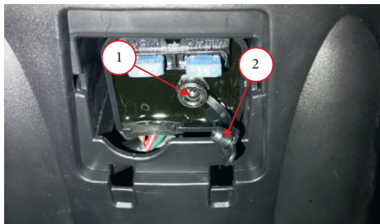
Фото 4. Место подключения зарядки АКБ: 1 – разъем для подключения зарядного устройства; 2 – колпачок.
