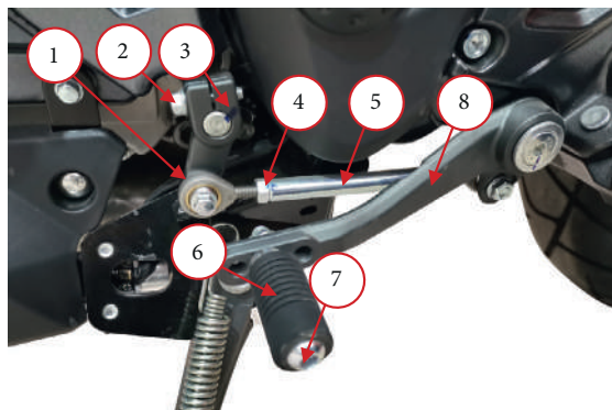
Фото 2.16. Регулировка рычага переключения передач:
