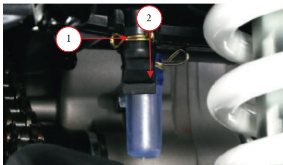
Фото 4.2. Слив загрязненного масла: 1 – крепежный хомут; 2 – трубка слива.
