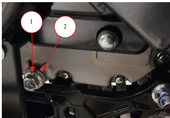
Фото 4.5. Слив моторного масла: сливной болт – 1; шайба – 2.
