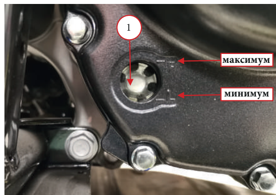
Фото 2.24. Контроль уровня масла:
