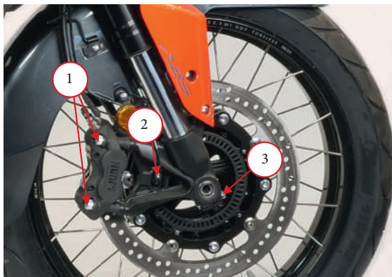
Фото 4.13. Снятие переднего колеса (вариант): 1 – болты тормозного суппорта; 2 – болт крепления датчика скорости; 3 – болт крепления оси.
