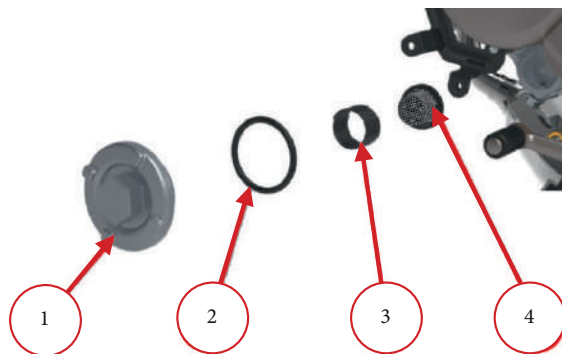
Фото 4.6. Снятие фильтра-сетки: 1 – крышка; 2 – уплотнительное кольцо; 3 – пружина; 4 – фильтр-сетка.
