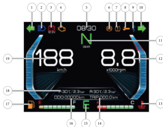
Фото 2.9. Приборная панель моделей ZT350-R/R1, ZT350-X/X1, ZT350-T, ZT350-GK, ZT350-VX, ZT350-V1, ZT350-S: 1 - индикатор левого поворота; 2 - индикатор дальнего света; 3 - индикатор напряжения аккумулятора; 4 - индикатор неисправности двигателя; 5 - часы; 6 - индикатор системы ABS; 7 - индикатор низкого давления в шинах; 8 - индикатор ТО; 9 - индикатор Bluetooth-подключения; 10 - индикатор правого поворота; 11 - текущая передача; 12 - тахометр; 13 - шкала температуры охлаждающей жидкости; 14 - текущий километраж; 15 - текущий режим (ЭКОНОМ/СПОРТ); 16 - общий километраж; 17 - шкала уровня топлива; 18 - температура воздуха/давление в шинах; 19 - спидометр.
