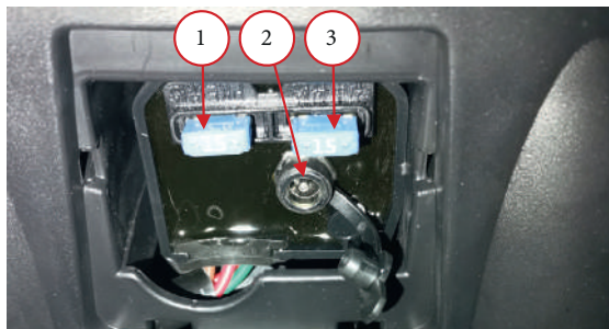
Фото 2.6. Элементы контроллера: 1 – предохранитель заряда АКБ; 2 – разъем для зарядки АКБ; 3 – предохранитель системы бесключевого доступа (номинал 15 А).
