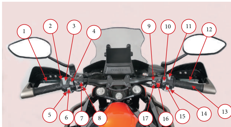
Фото 2.1. Вид руля и органов управления мотоцикла (с бесключевым доступом):
