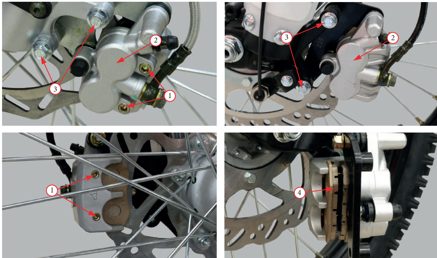
Фото 5.24. Замена передних тормозных колодок
